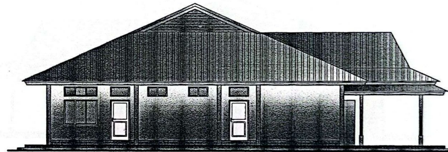
TAMPAK SAMPIING KANAN SKALA 1 : 100
