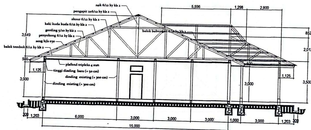
POTONGAN B SKALA 1: 100
