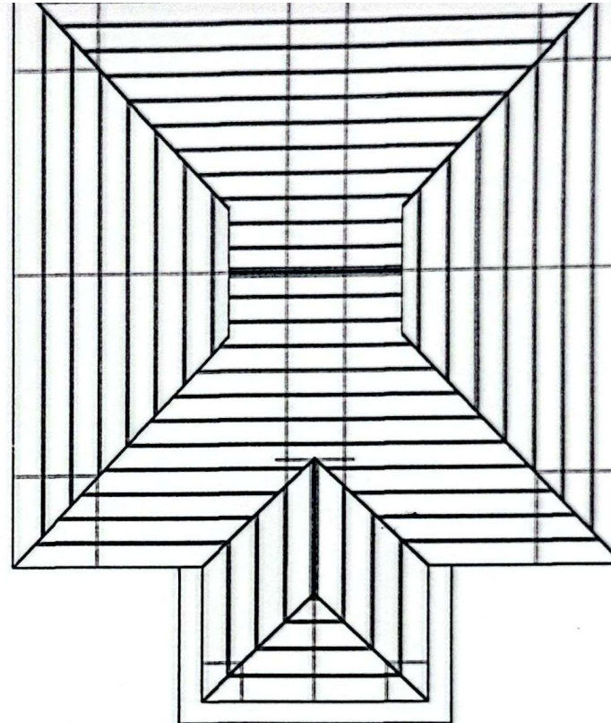
KUDA - KUDA ATAP SKALA 1 : 100
