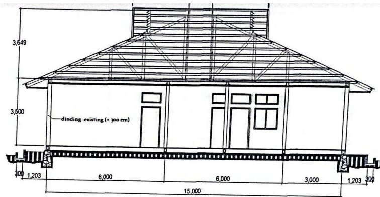
POTONGAN A SKALA 1: 100
