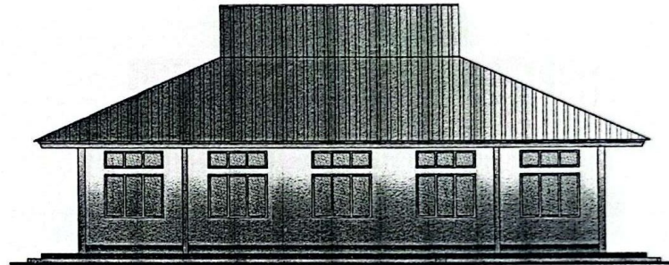
TAMPAK BELAKANG SKALA 1 : 100
