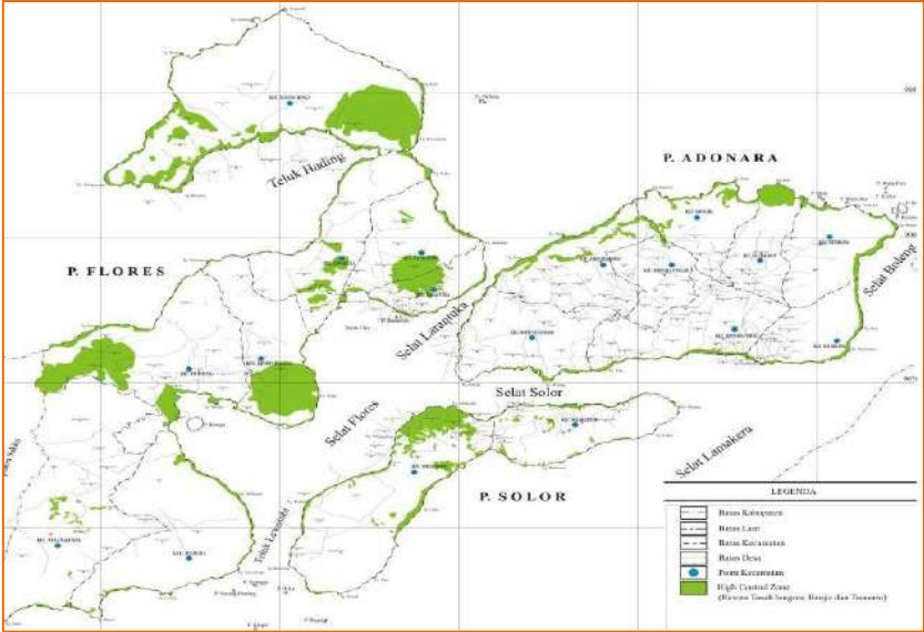
Gambar 2.2 Peta Zona Rawan Tanah Longsor, Banjir dan Tsunami (sumber: RTRW Kab. Flotim Tahun 2007-2027)
